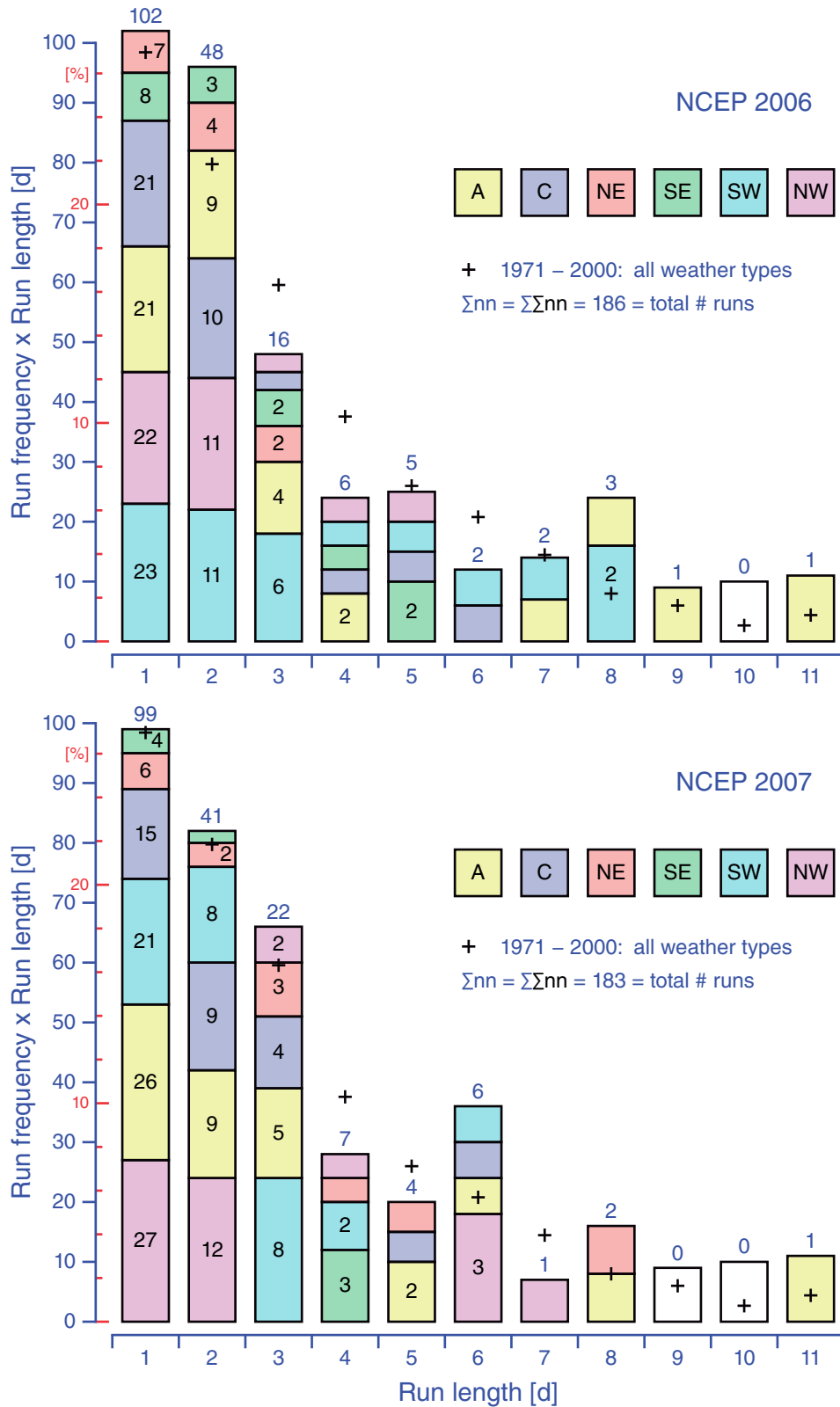
Abb. 2-6: Skalierte Histogramme (gestapelt) für die Lauflänge (rl) der Wetterlagen (w) in den Jahren 2006 & 2007. Basis %-Skala: 365 Tage. Höhe Stapelelemente: rl × Anzahl Läufe r(w,rl). Schwarze Zahlen: r(w,rl), blau: r(rl). + Symbole: rl × r(rl) × 365/10958 d für 1971 – 2000.
