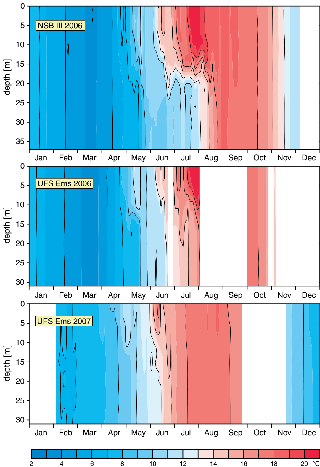
Abb. 3-19: Temperaturschichtung (°C) an den MARNET-Stationen »NSB III« (54° 41' N, 6° 47' E) und »Ems« (54° 10' N, 6° 21' E). Wasser- und Sensortiefen: 40 m & 4, 6, 11, 15, 20, 25, 30, 35 m und 33 m & 3, 6, 10, 15, 20, 25, 30 m.
