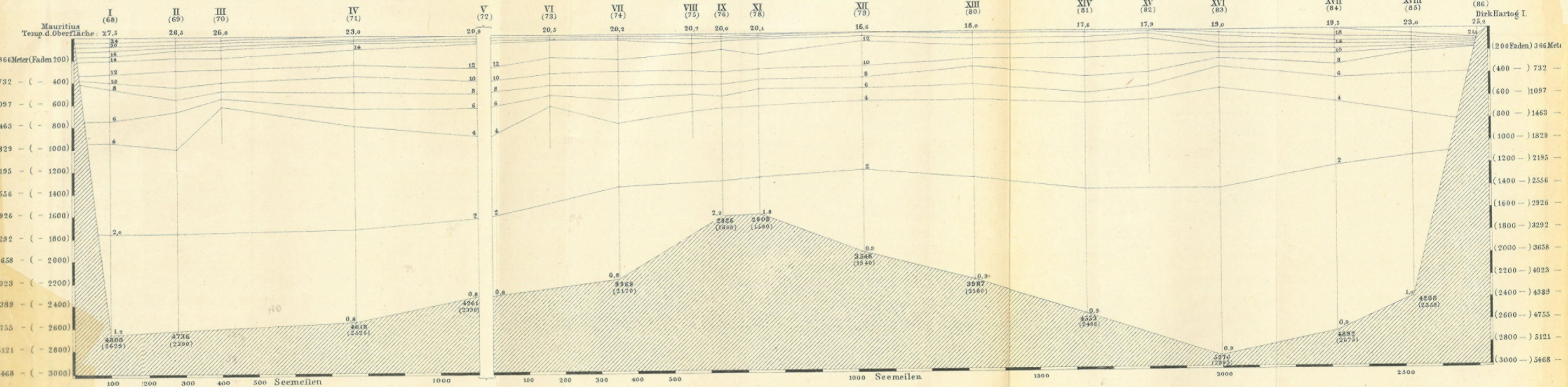
Diagramm II. Isothermen zwischen Mauritius und Dirk Hartog I, West-Australien.
