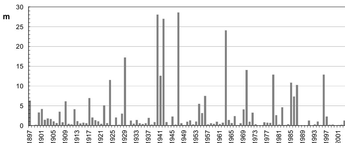
Abbildung 5.4. Flächenbezogene Eisvolumensumme ( V_{A\Sigma} ) für die deutsche Ostseeküste im Zeitraum 1897-2004 Figure 5.4. Accumulated areal ice volume ( V_{A\Sigma} ) for the German Baltic Sea coast in the period 1897-2004
