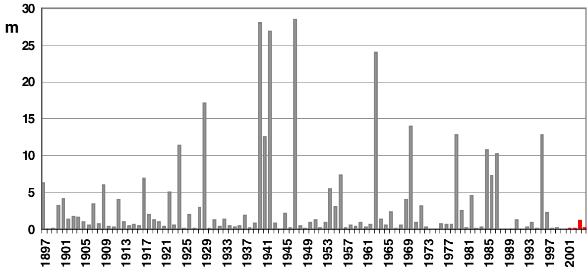
Flächenbezogene Eisvolumensumme für die deutsche Ostseeküste Accumulated areal ice volume for the German Baltic Sea coast
