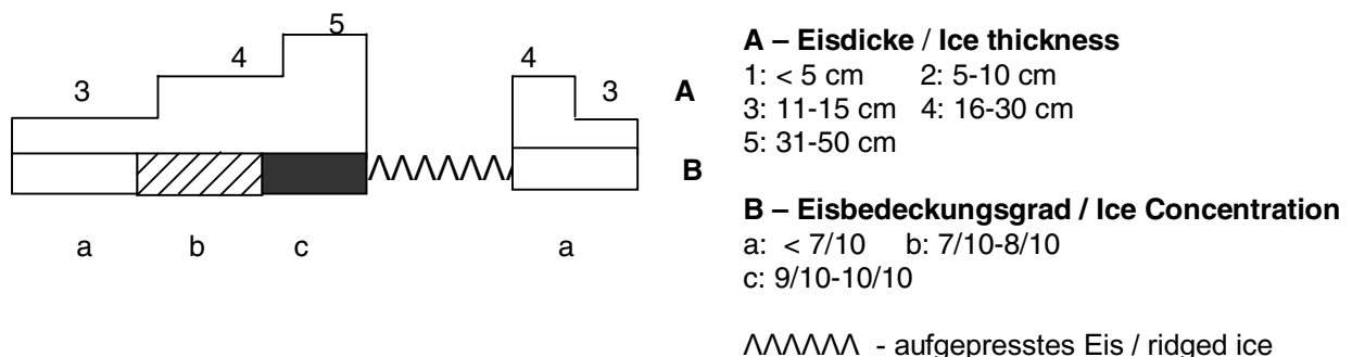
Abbildung 1.3. Bedeckungsgrad und Dicke des Eises in den Fahrwasserabschnitten und Häfen an der deutschen Ostseeküste im Winter 1999/2000 Figure 1.3. Ice concentration and thickness in the fairways and harbours of the German Baltic coast in the winter of 1999/2000
