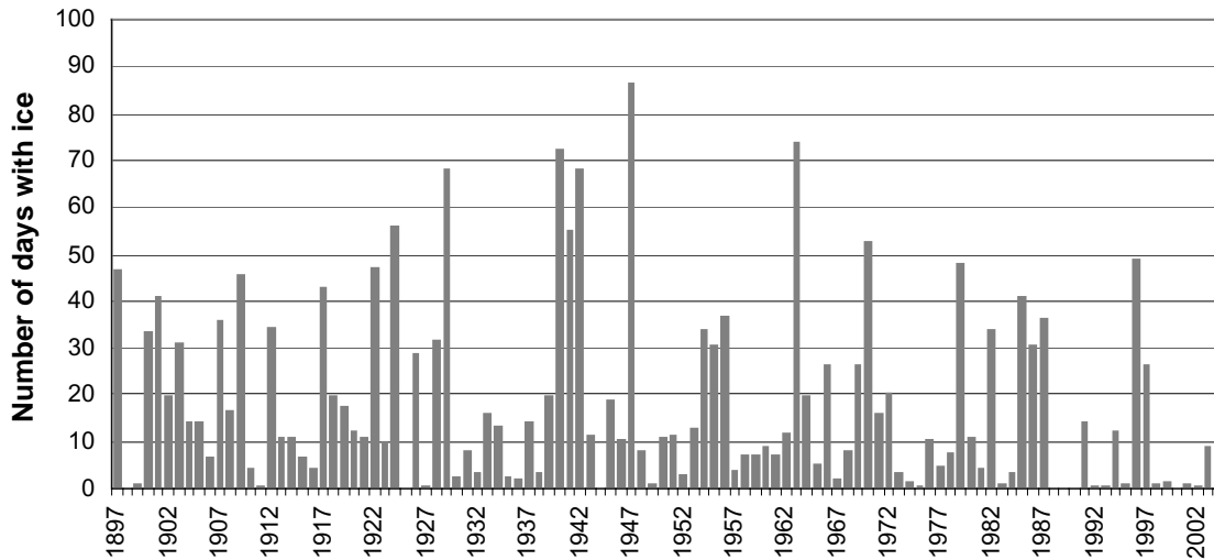
Abbildung 5.1. Reduzierte Eissumme für die deutsche Nordseeküste im Zeitraum 1897-2004 Figure 5.1. Reduced sum of ice for the German North Sea coast in the period 1897-2004
